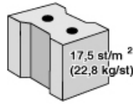
BIA 26-24 klinker LxBxH = 220x265x240 (38,0 ltr specie per m 2 )
