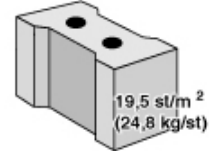
BIA 32-24 klinker LxBxH = 200 x 320 x 240 (47,5 ltr specie per m 2 )
