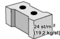
BIA 32-19 klinker LxBxH = 200x320x190 (60,5 ltr specie per m 2 )
